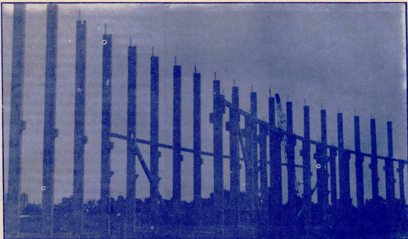
Plano general de la Tribuna Oeste con todas las columnas colocadas.
