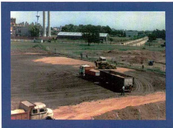
Los camiones trabajan para nivelar el sector del campo de juego, el cual contará con ocho canales para el drenaje y pequeños afluentes en cada uno de ellos.
